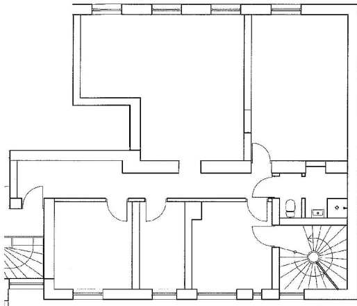
Plantegning
