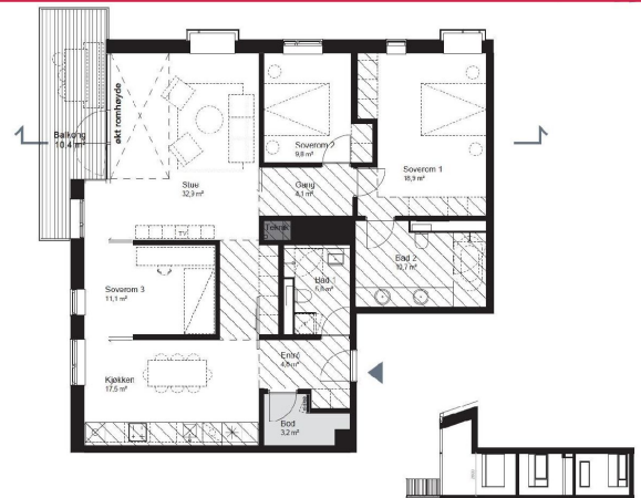
Plantegning
