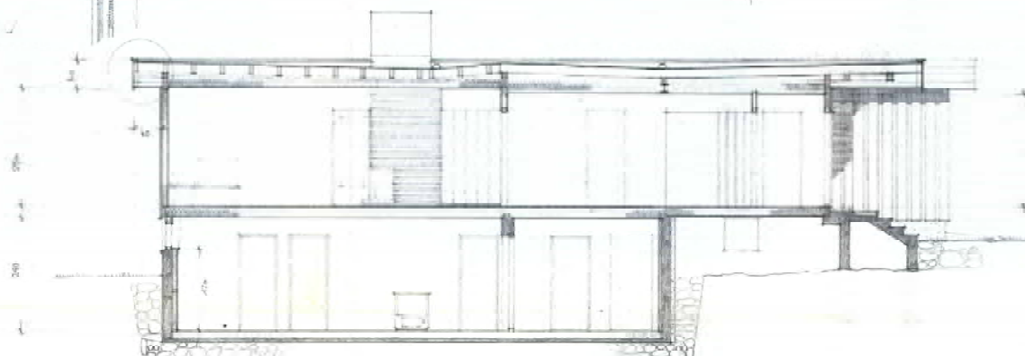
SNITT A-A
