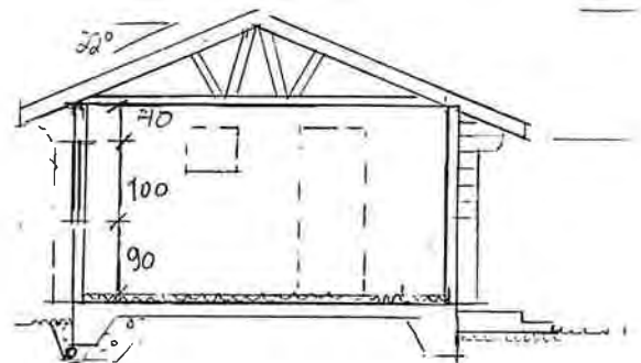
SNITT
