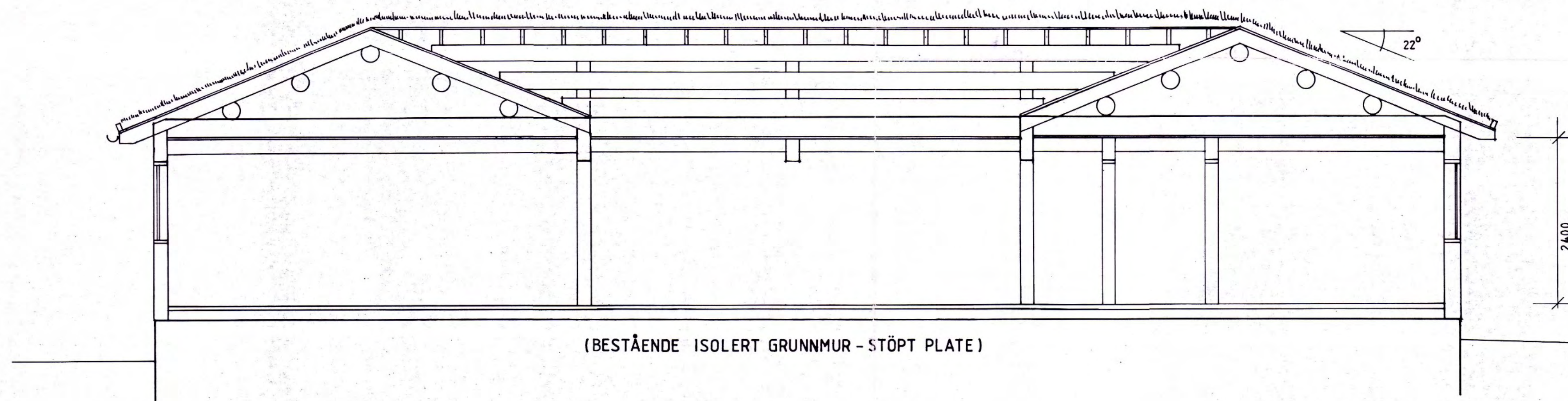
SNITT A-A
