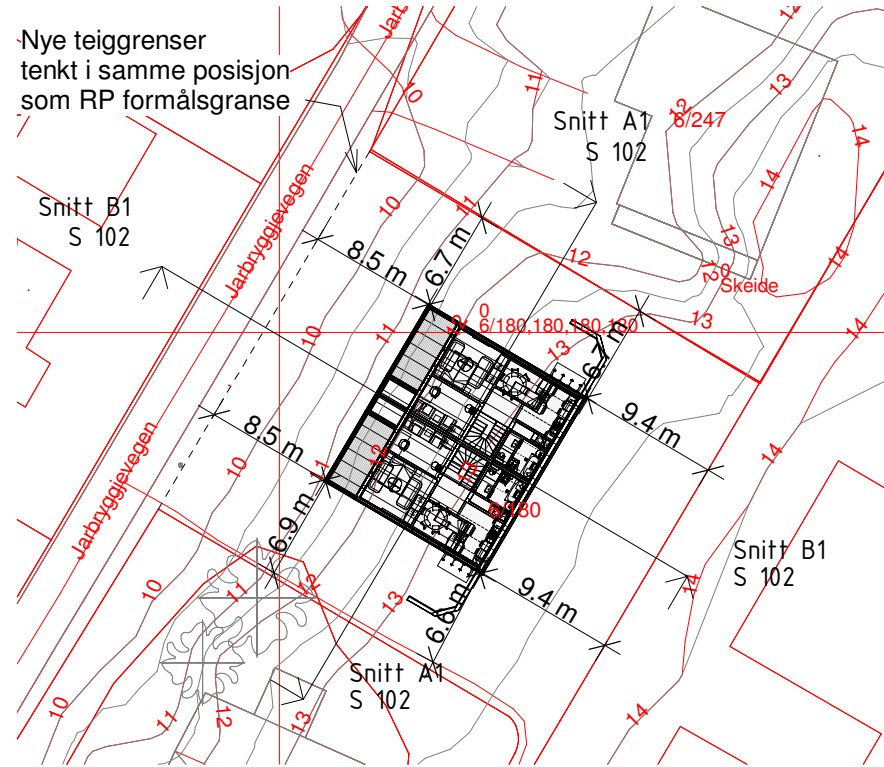
Situasjonsplan 1 : 500
