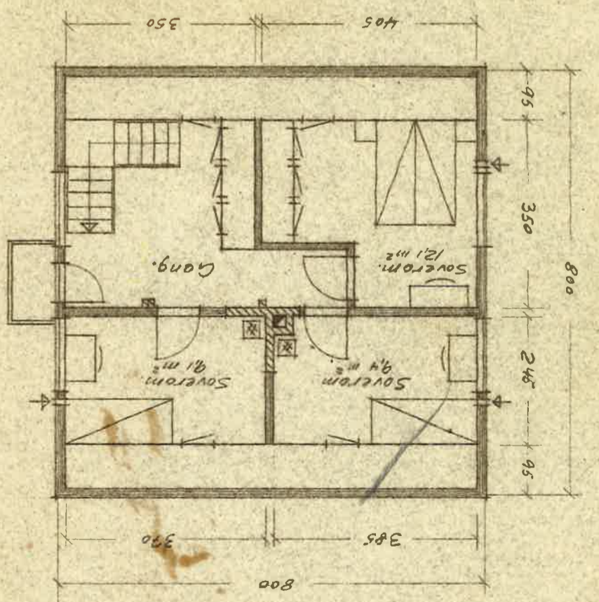
2. etasje. Learea = 47 m 2
