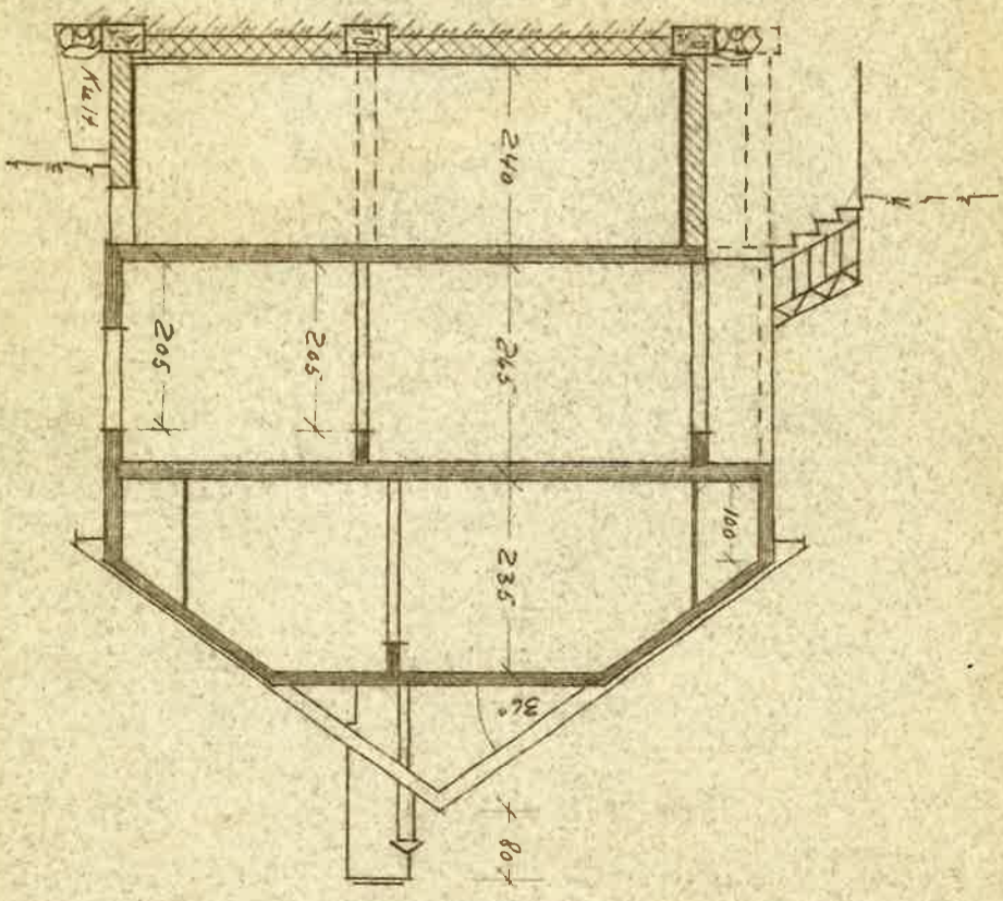
Snitt A.
