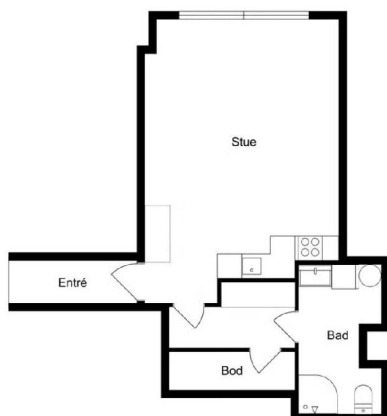
Plantegning
