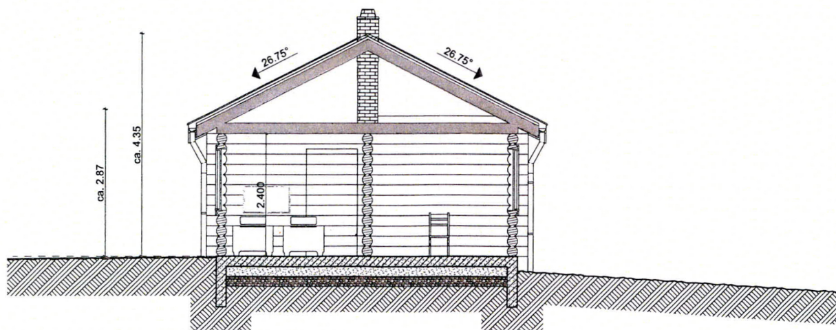
Snitt AA
