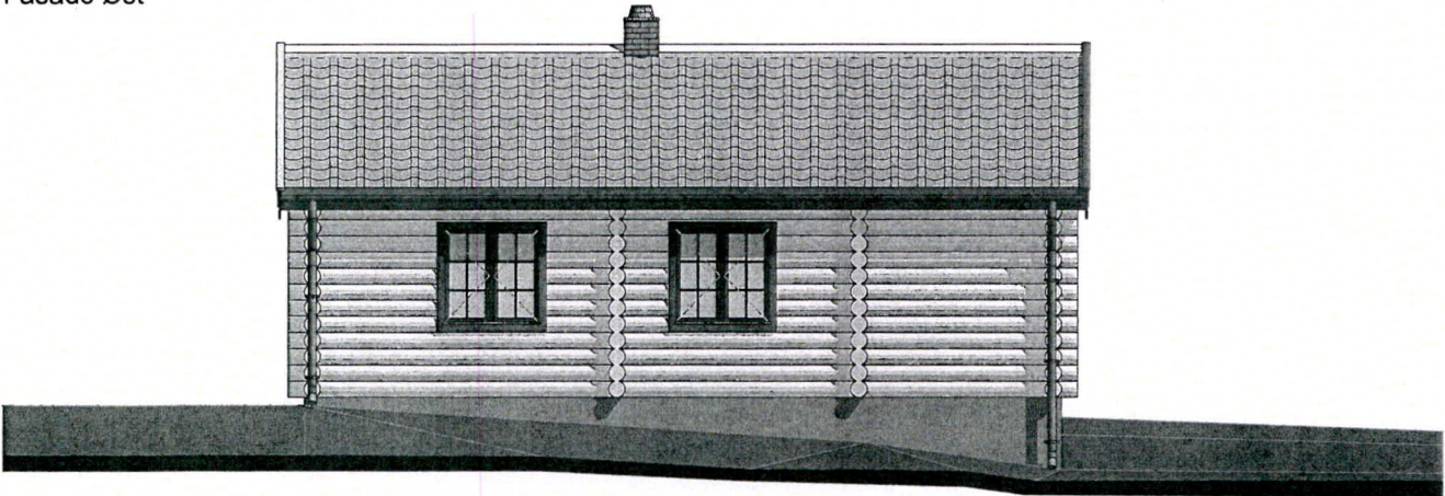
Fasade Øst
