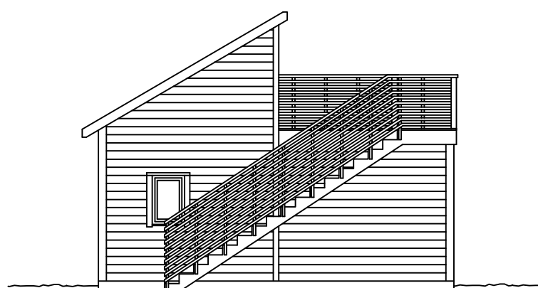
Garasje Fasade mot Nord
