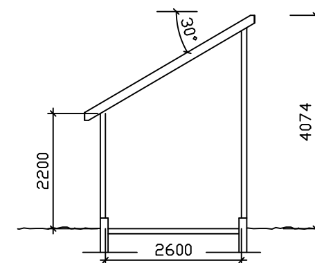
Bod Snitt
