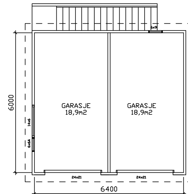
Garasje Plan
