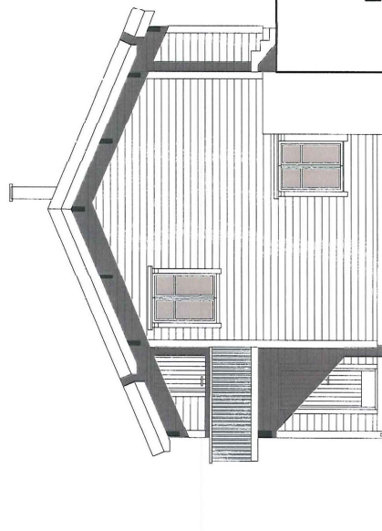
FASADE MOT Nor M=1:100
