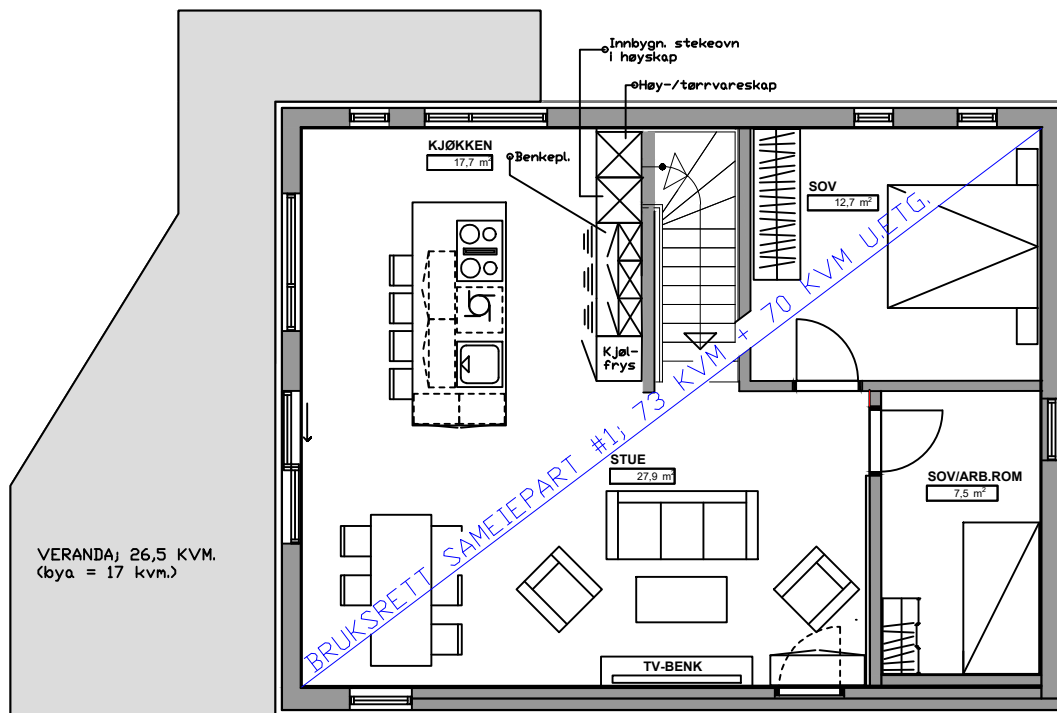
HOVEDETASJE; 73 kvm
