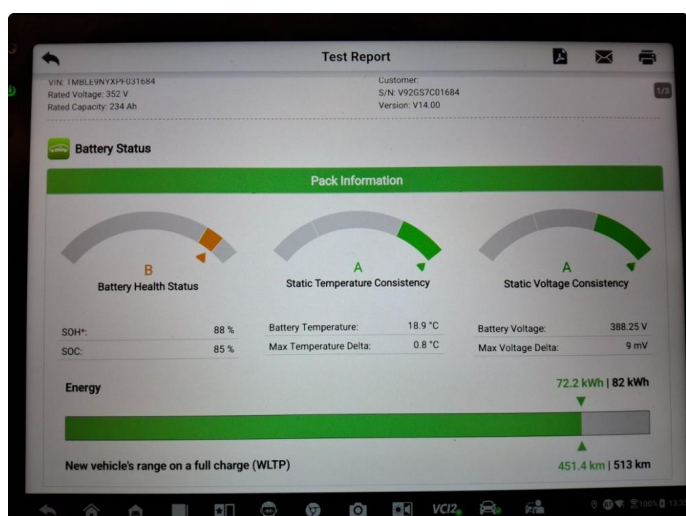
2.1 Batteritest
