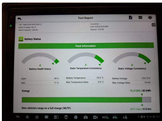
1.1 Batteritest
