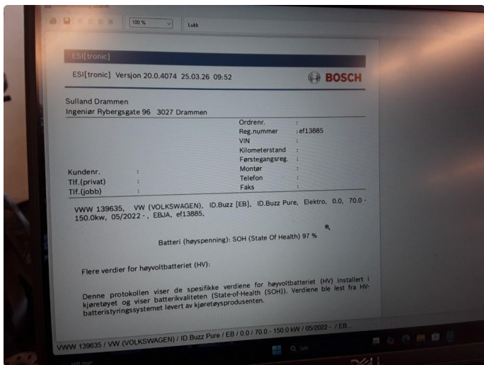
3.1 Batterikapasitet på 97 %
