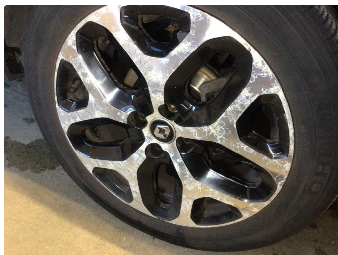
1.1 Noe oksidering på sommerfelger og en kantkjørt vinterfelg
