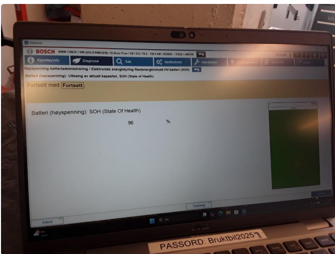
2.1 Batterikapasitet på 96%
