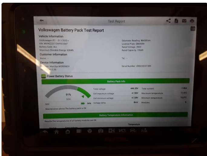
3.1 Batteri 91% SOH
