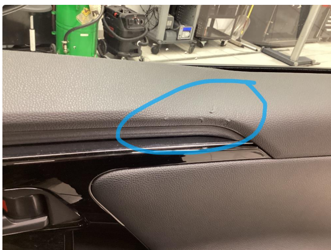
2.1 Rift
