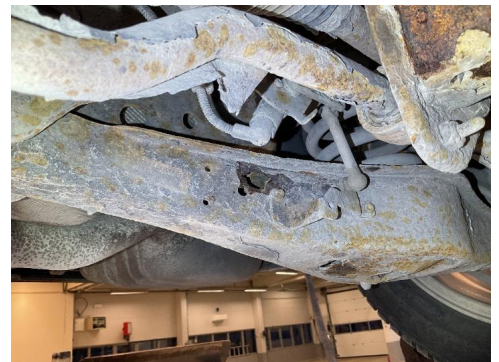
72. Opphengs- / bærearmer bakaksel
