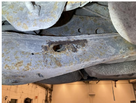
71. Opphengs- / bærearmer bakaksel
