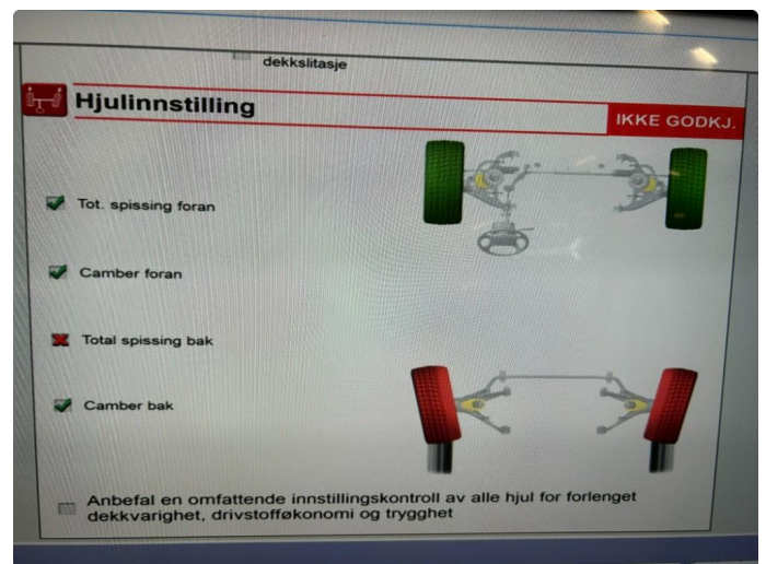
3.1 4-hjulsmåling/forstillingskontroll (utføres)
