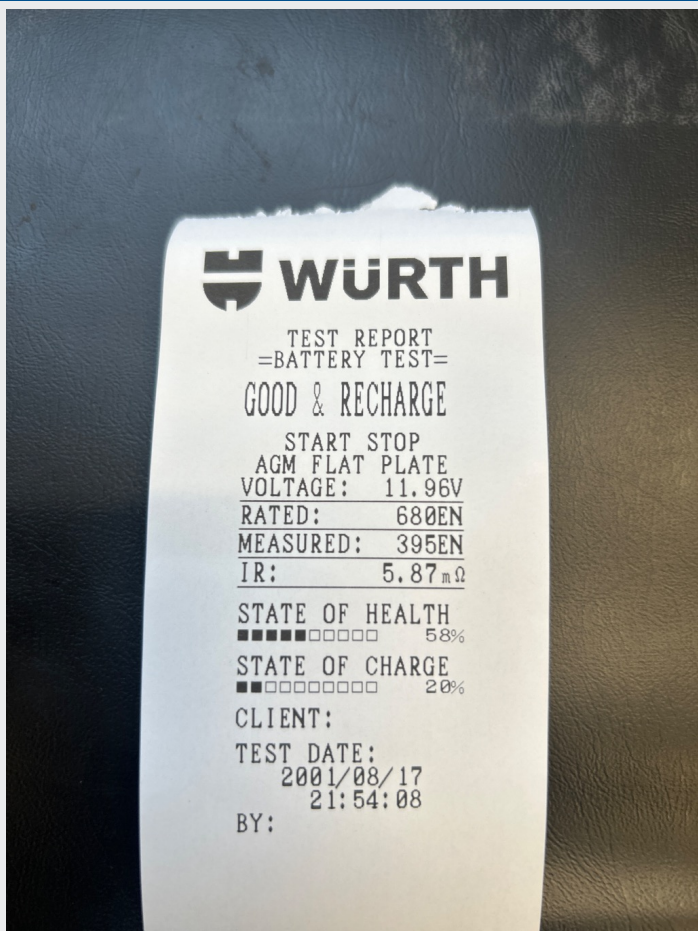
5.2 Batteritest
