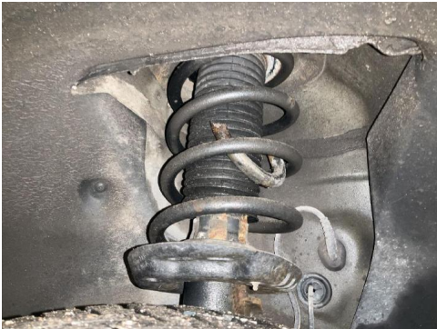
37. Fjærer / fjærbein
