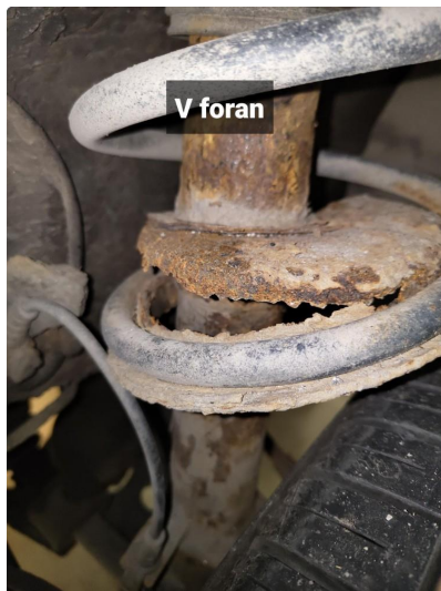
4.1 Demperskål, gjennomrustet og bøyd/skadet
