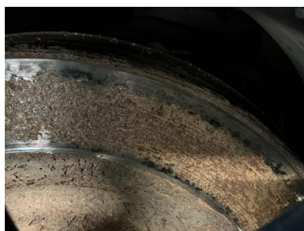
6. Bremseskiver
