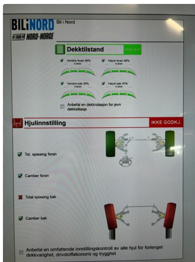
3.1 4-hjulsmåling/forstillingskontroll
