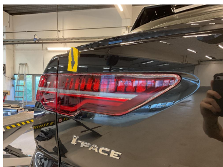
31. Lys
