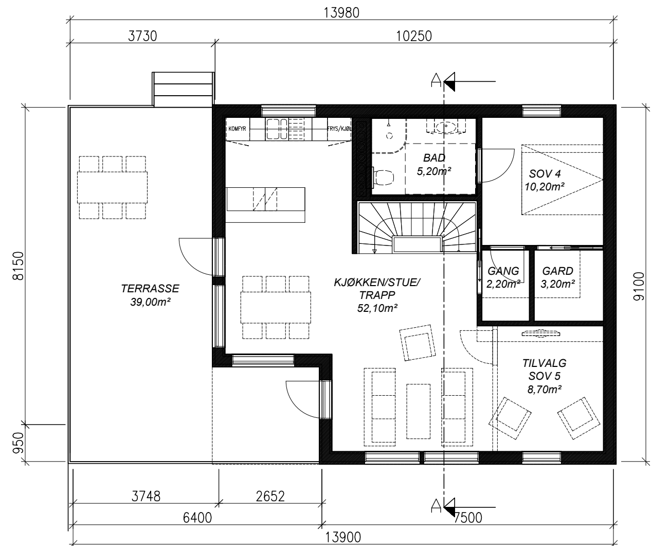
PLAN 2.ETG
