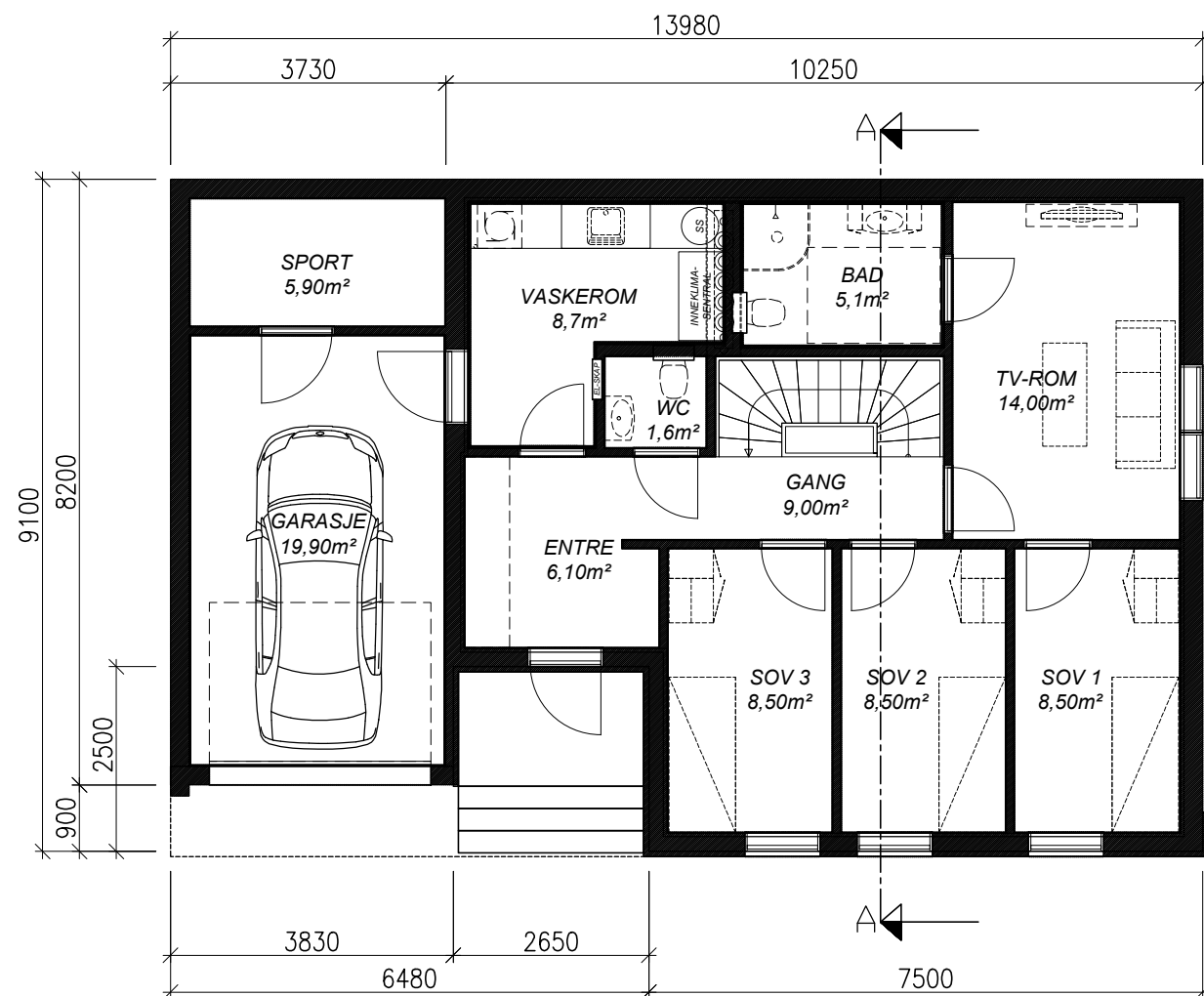
PLAN 1.ETG
