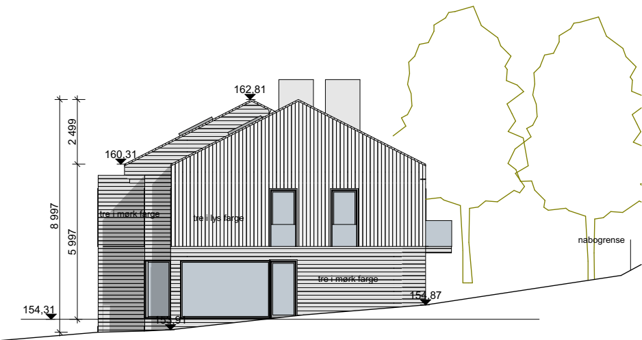
Fasade vest Hus B
