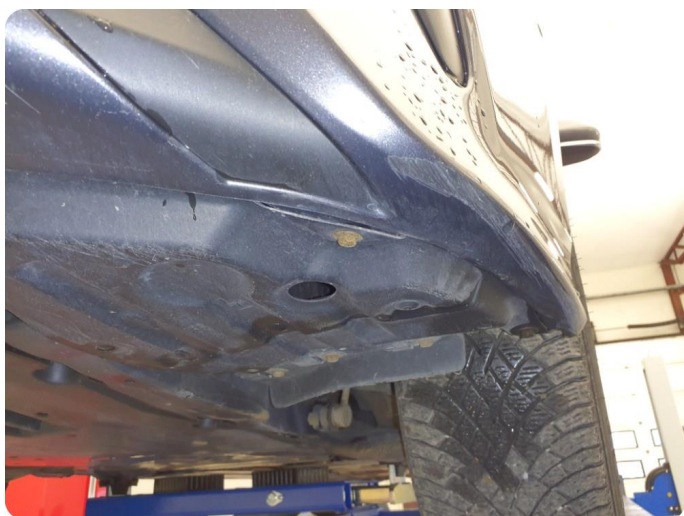
2.9 Skrubbskader underkant
