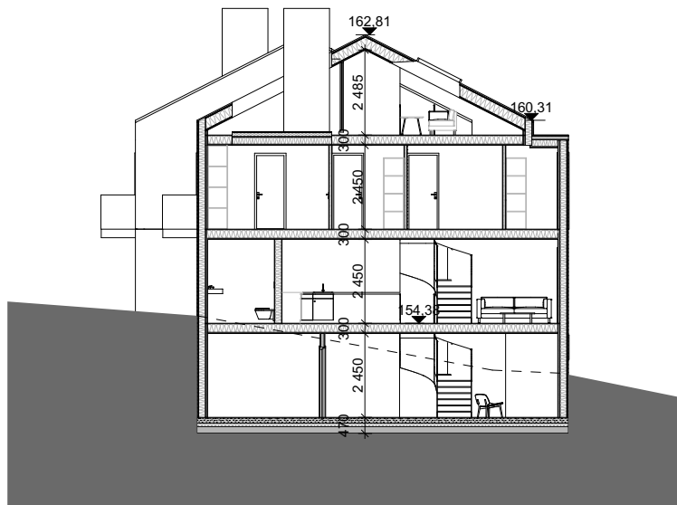
Snitt B
