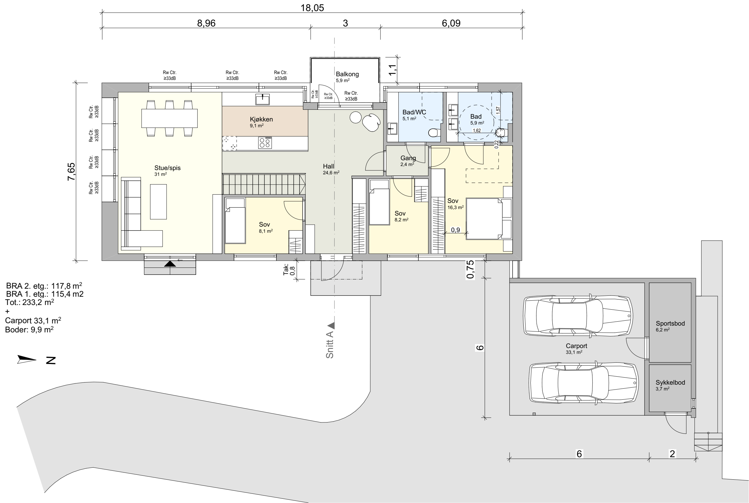
2. etasje Hus B
