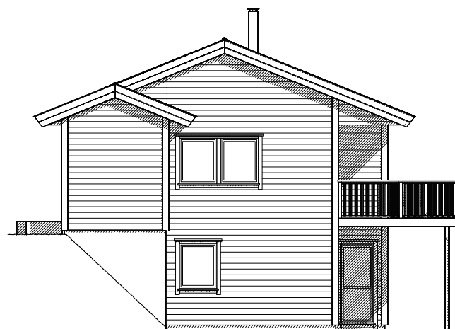
FASADE MOT SØR-VEST
