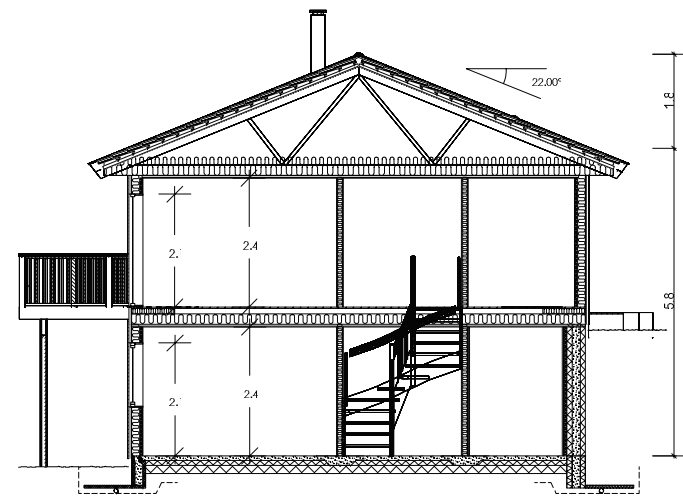
SNITT A-A
