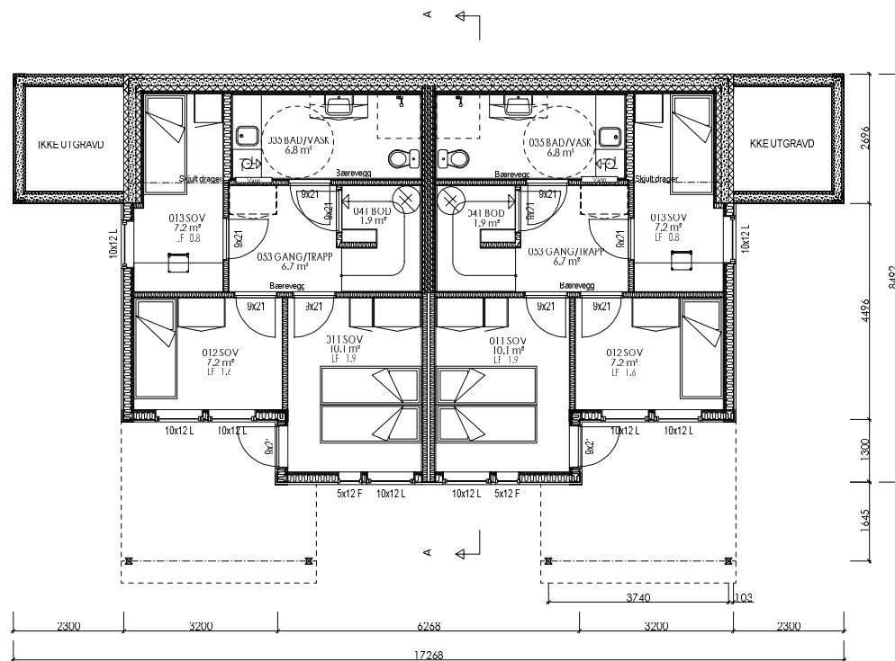
SOKKELPLAN
