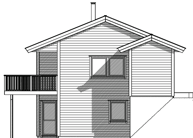
FASADE MOT NORD-ØST
