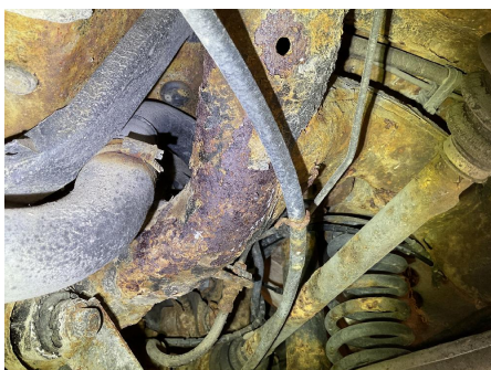
41. Travers
