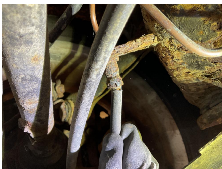
50. Bremseslanger
