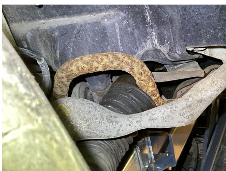
56. Styresnekke, tannstang
