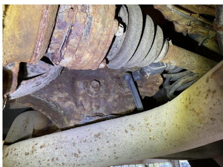
43. Travers
