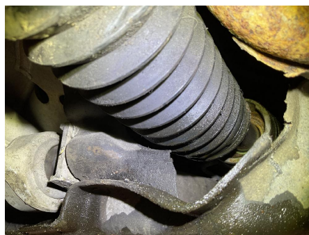
39. Styresnekke, tannstang
