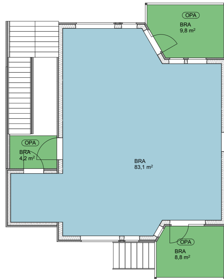
1:120 BRA 1. etasje
