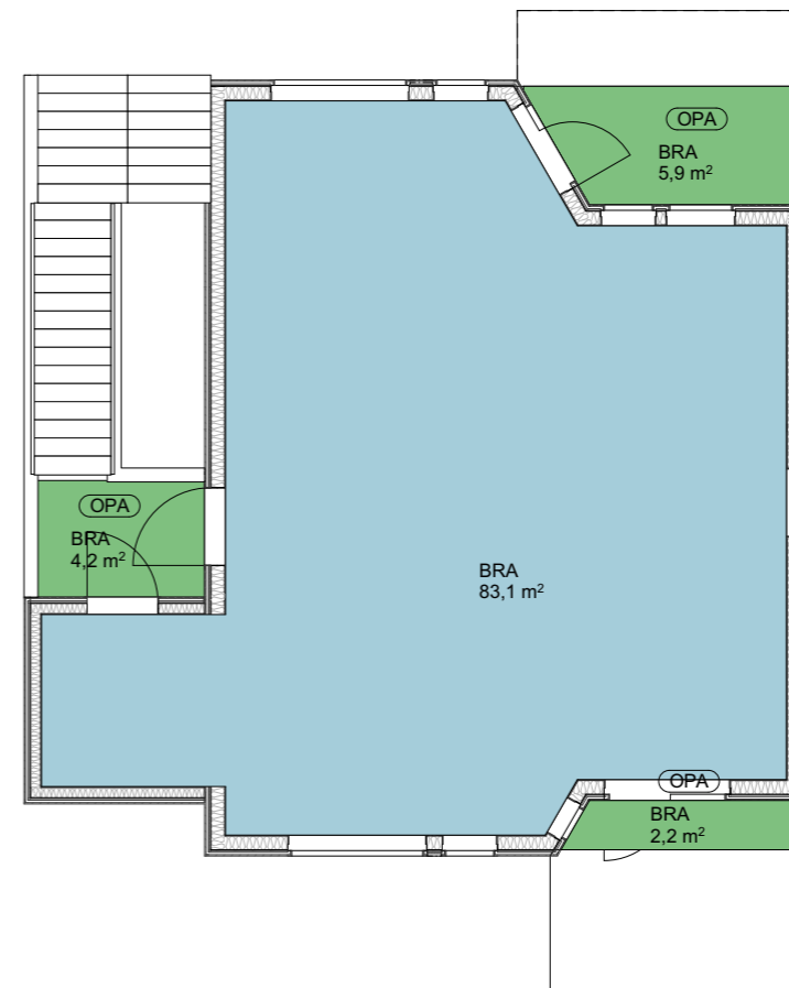
1:120 BRA 2. etasje
