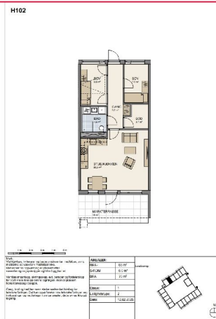
Plantegning H102
