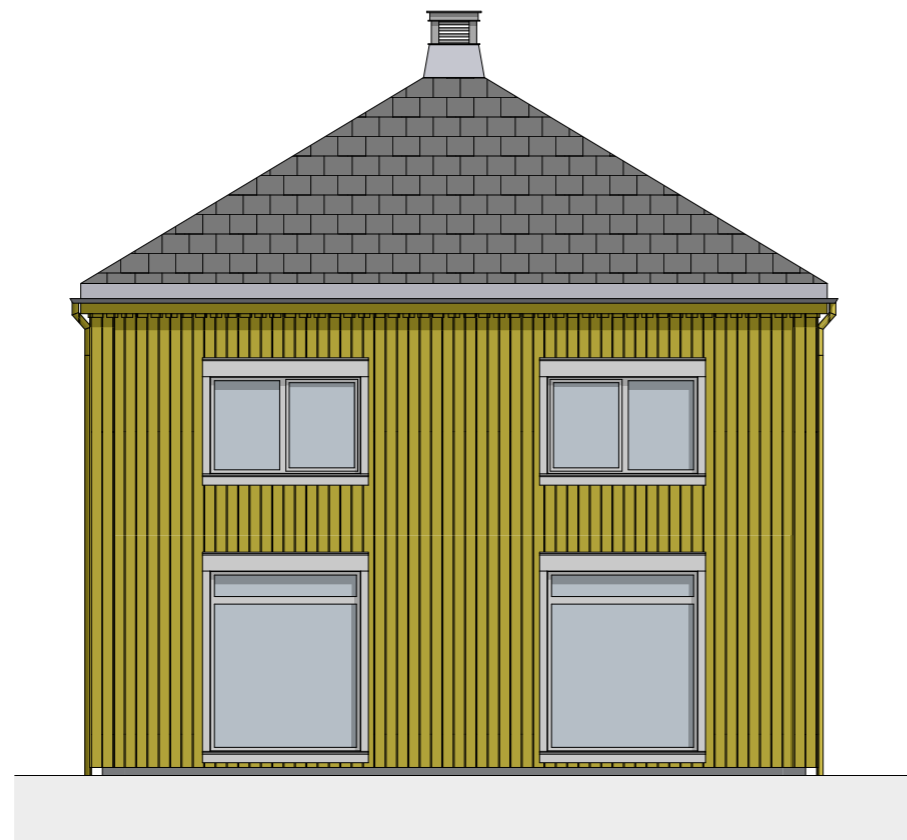
Fasade Sørvest 1:100
