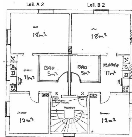
Plategning. Leilighet venstre er vendt ut mot Bergensgata, leilighet høyre er vendt mot bakgård/gate
