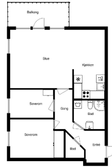
Plantegning
