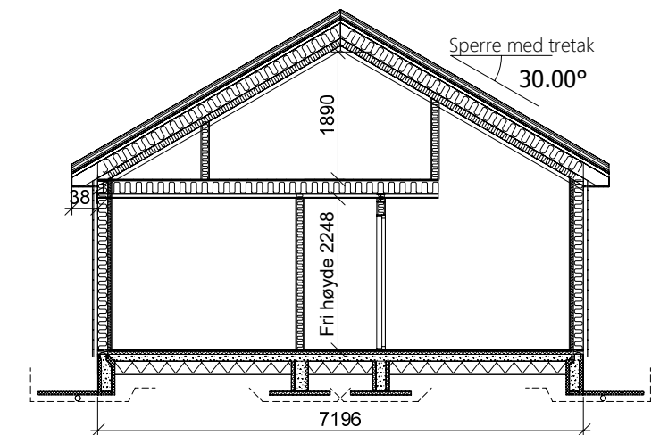
SNITT A-A
