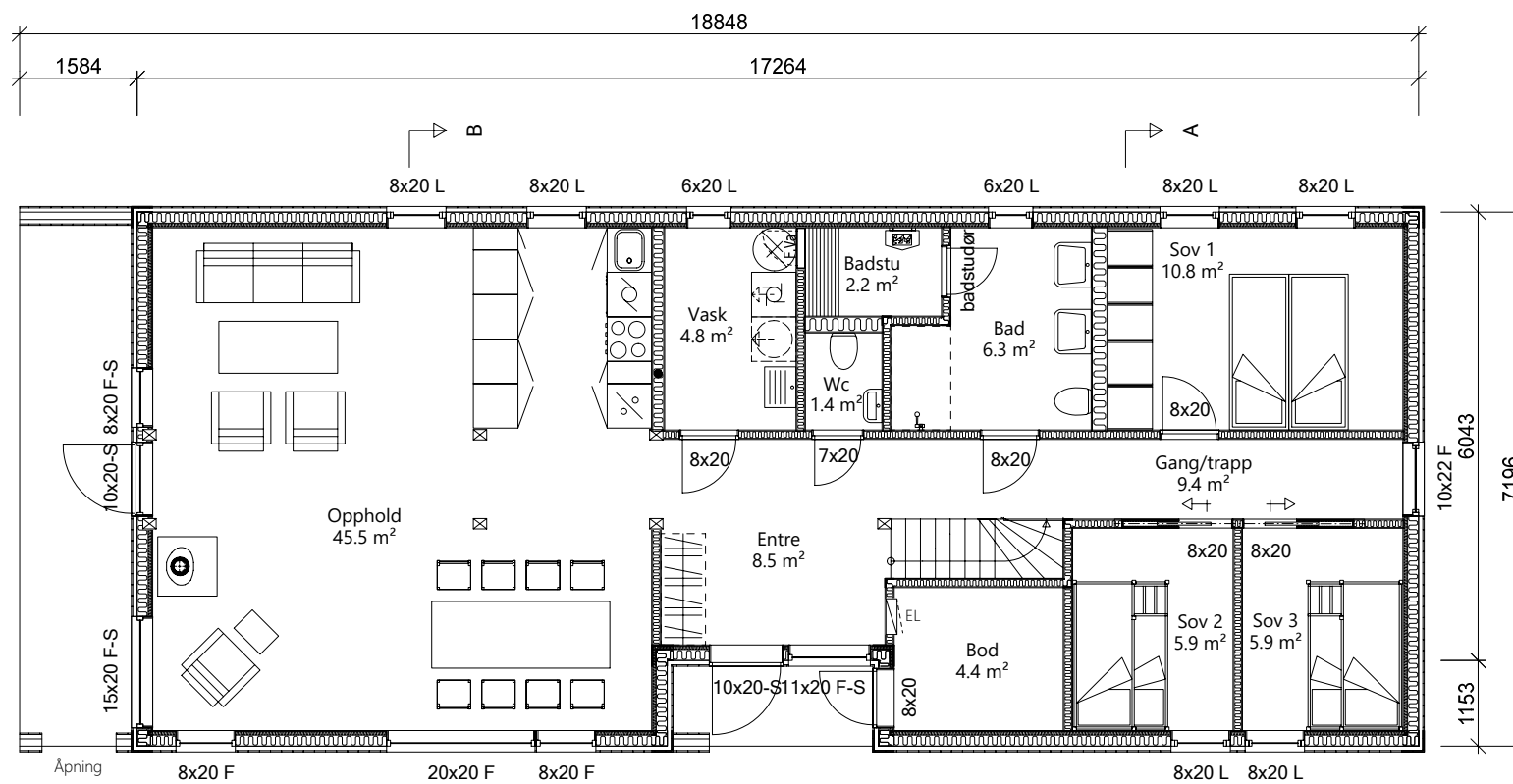
PLAN 1.ETG
