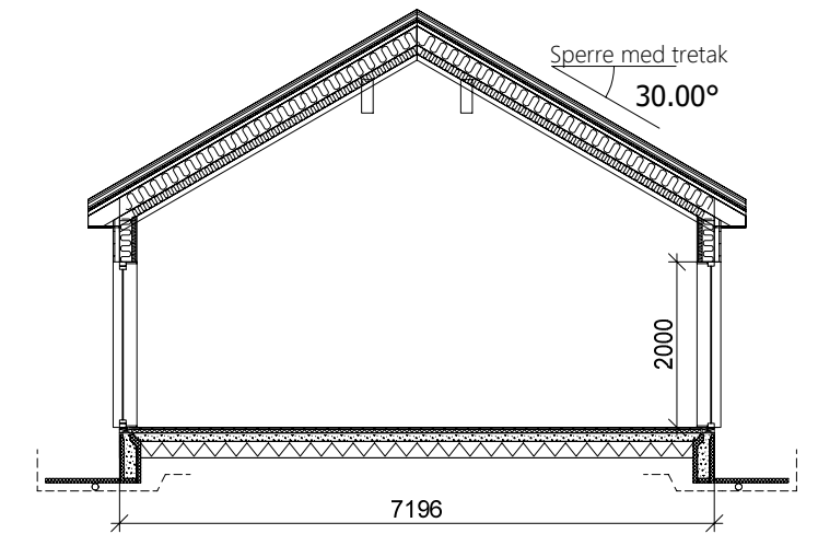
SNITT B-B
