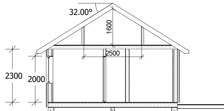
Snitt A-A
