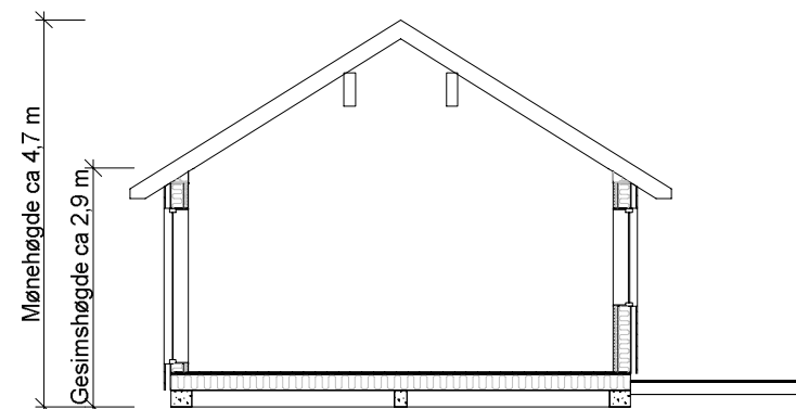
Snitt B-B
