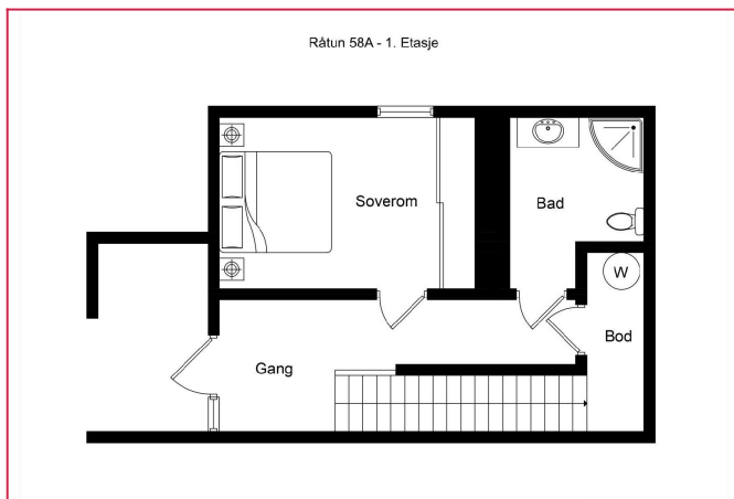
Plantegning 1.etg.
