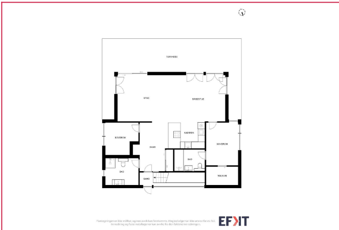
Planskisse 1. etasje
