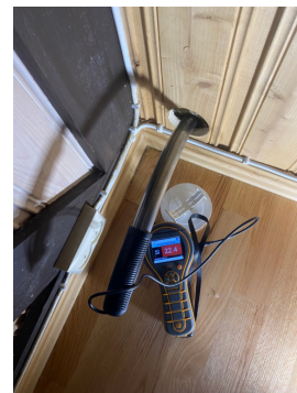
Fuktmåling i vegg i kjellerstue med forhøyde verdier.
