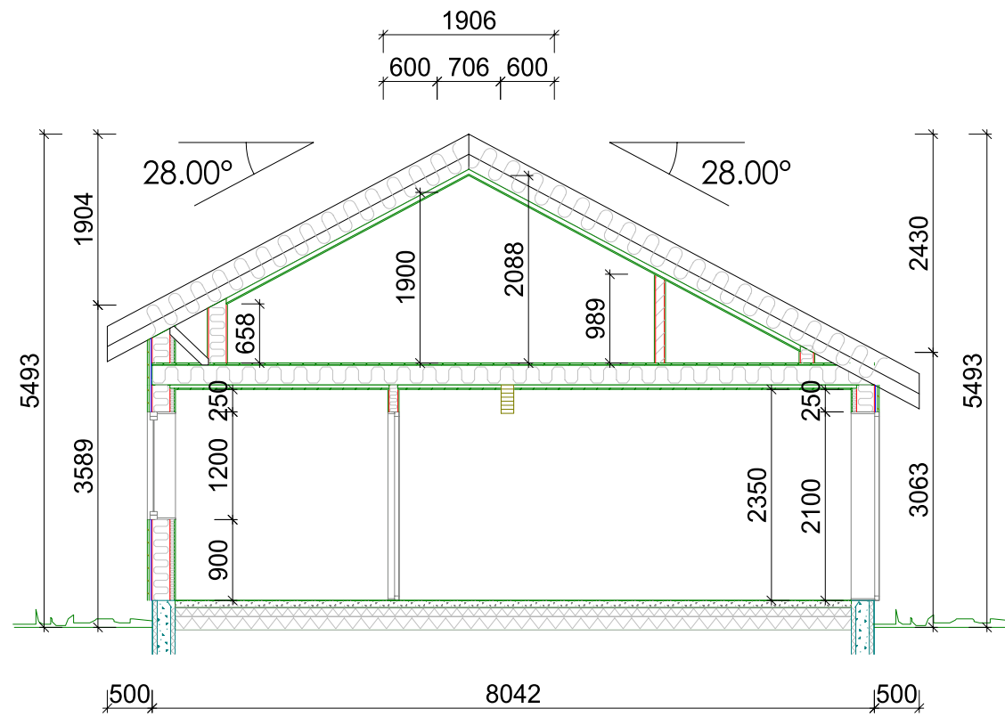
Snitt A-A
