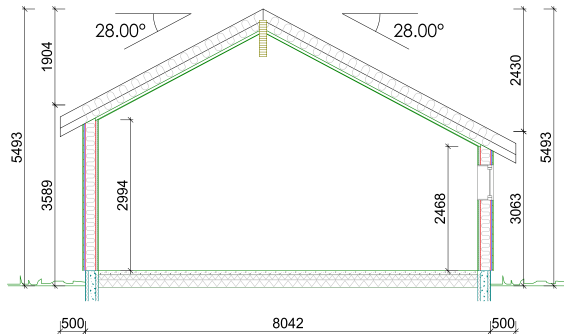
Snitt B-B
