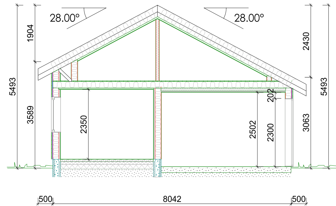
Snitt C-C
