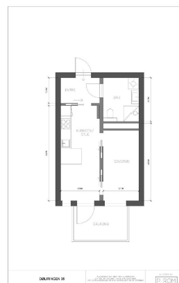
Plantegning
