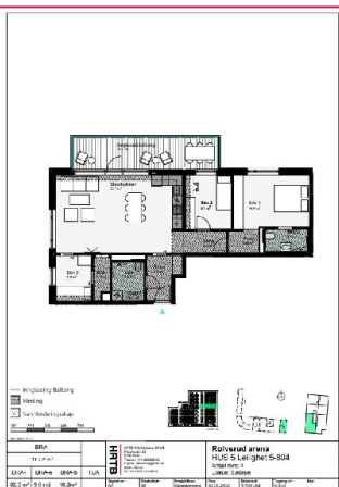
Plantegning 5-804
