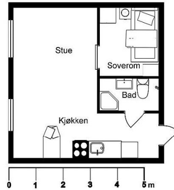
Planskisse
