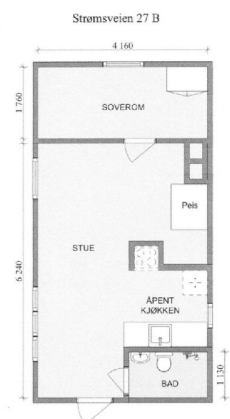
Plantegning
