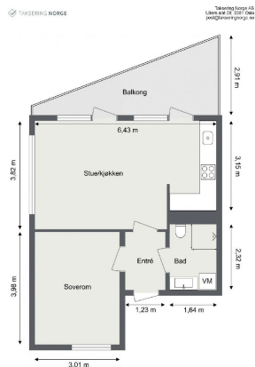
Plantegning
